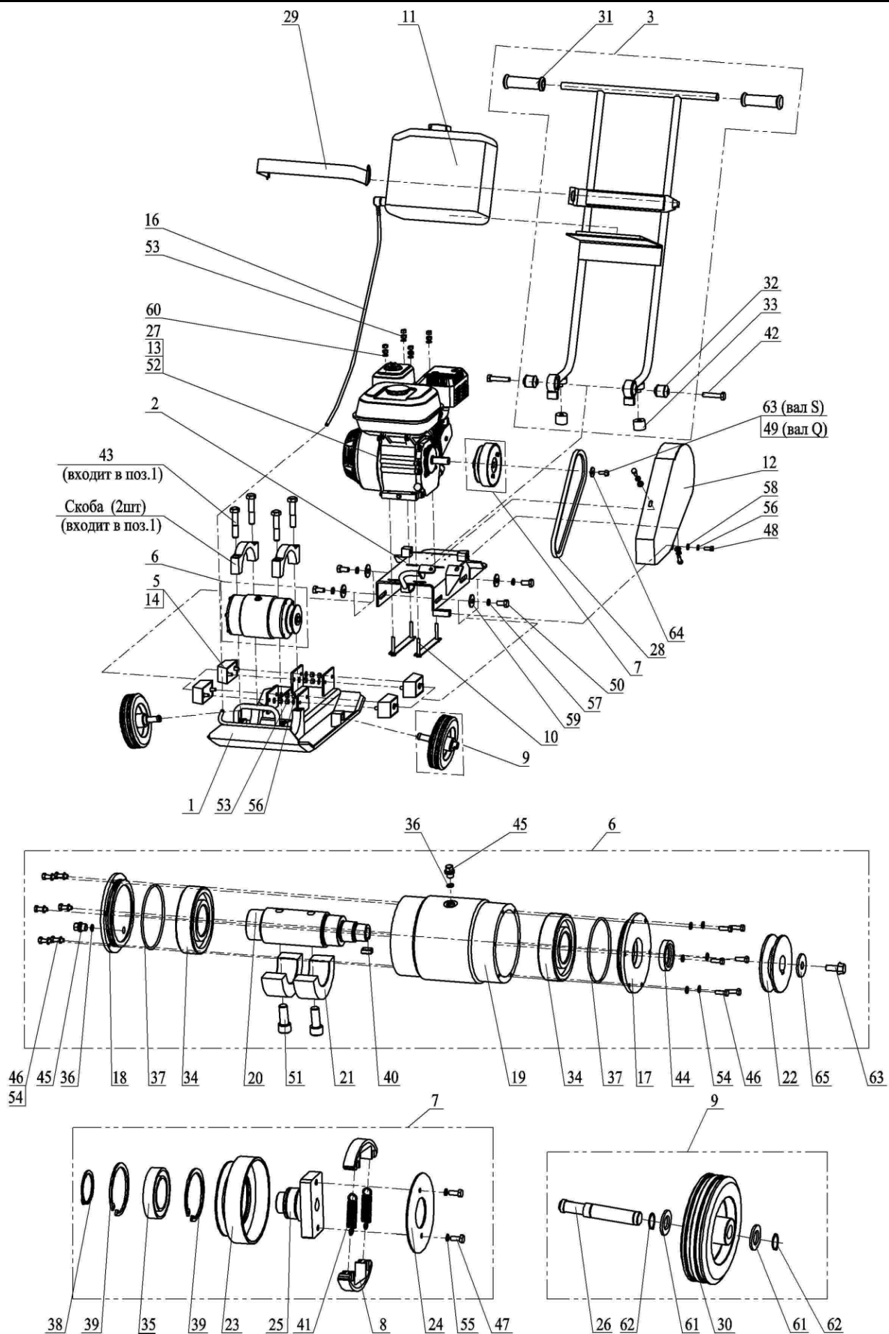
Рисунок 8 – Компоновка виброплиты
